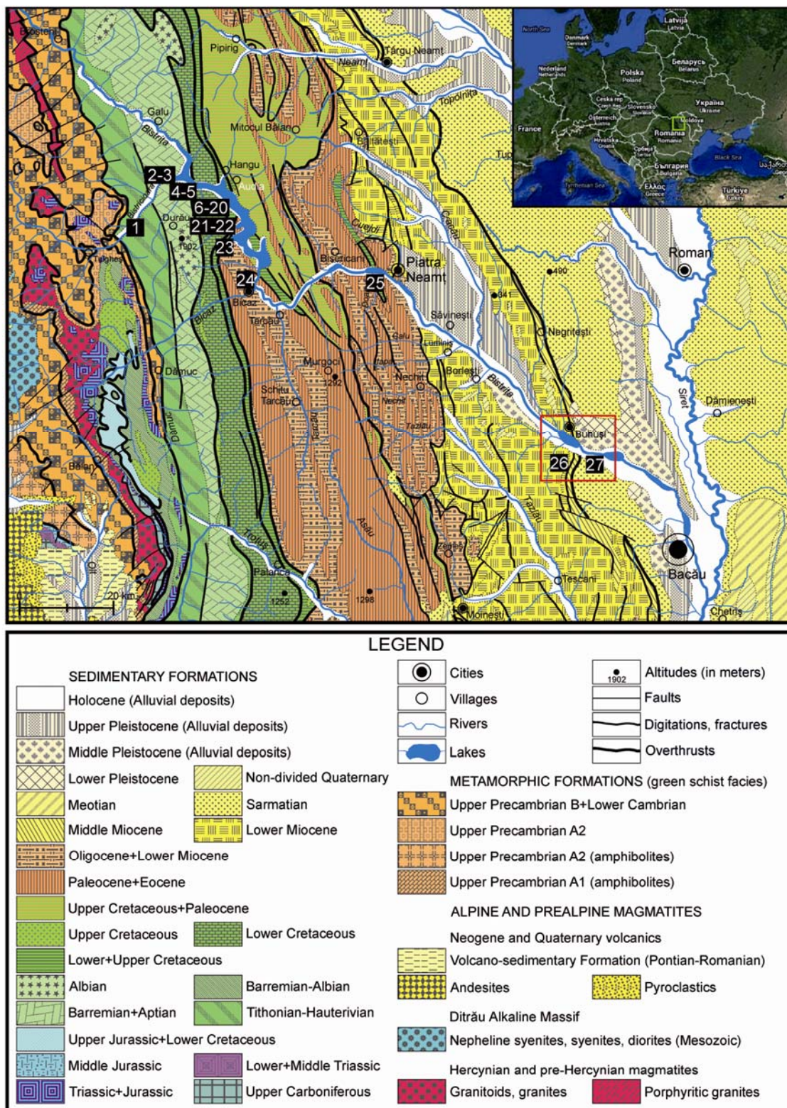
Plate 1. Location and geological context of Upper Palaeolithic sites from the Middle and Lower Bistrița Valley: 1. Bradu-Pârâul lui Oloi La Râpă; 2.-3. Grințieș-Frasinu I-II; 4. Bistricioara-Lutărie; 5. Bistricioara-Lutărie La Mal; 6.-7. Ceahlău-Cremenii I-II; 8. Ceahlău-Bofu Mic; 9. Ceahlău-Bofu Mare; 10.-13. Ceahlău-Cetățica I-IV; 14. Ceahlău-Curtea Bisericii Vechi; 15. Ceahlău-Dârțu; 16. Ceahlău-Schitisor; 17. Ceahlău-Palatul Cnejilor; 18. Ceahlău-Lutărie; 19. Ceahlău-Podiș A-B; 20. Schitu-Curtea Bisericeștei de lemn Schitisor; 21. Izvorul Alb-Culmea Baicului; 22. Izvorul Alb-Piciorul Gol; 23. Secu-Curtea Boului; 24. Bicaș-Ciungi; 25. Piatra Neamț-Poiana Cireșului; 26. Buda-Dealul Viilor; 27. Lespezi-Lutărie; mapping of sites has been done after Păunescu 1998 and Steguweit et alii 2009; map support was redrawn and modified after a part of the Geological Map of Romania 1: 1000000 (Săndulescu et alii 1978).
