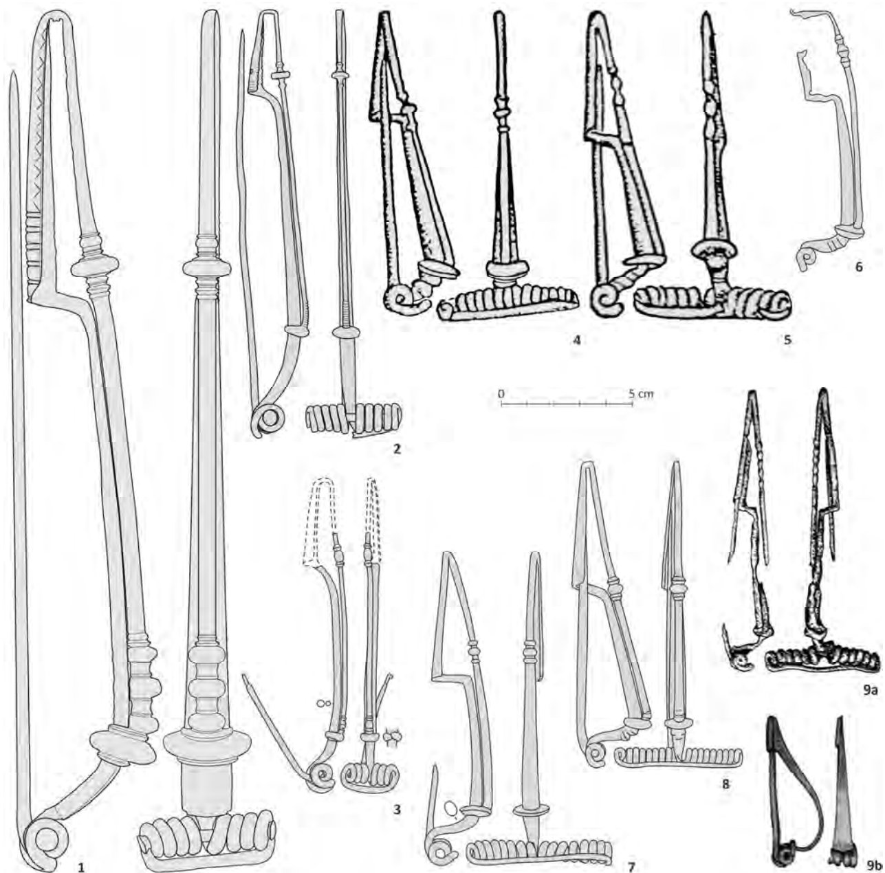
Figura 11. Fibule de schemă La Tène mijlociu cu perla încadrată de piruete pe picior (1–9a). 1. „Transilvania”; 2. Corlate, mormântul 1; 3. Desa, mormântul 12; 4. Sofronievo, mormântul 4; 5. Sofronievo, mormântul 5; 6. Pavolce, Ulovica, descoperirea 4; 7. Gura Padinii (scară ipotetică); 8. Pleven; 9a–b. Dobrești, locuință adâncită incendiată; 1–3. După original; 4–5. După Nikolov 1981, fig. 5a, 6b; 6. După Nicolov 1965, fig. 18g; 7. După Nicolăescu-Plopșor 1945–1947, fig. 4; 8. După Popov 1928–1929, p. 279, nr. 9, fig. 1/1–2; 9a–b. După Gherghe 1999, fig. 1/2–3. 1. Argint; 2, 4–5, 8, 9a–b. Fier; 3, 6–7. Bronz / Fibulae of Middle La Tène scheme with the motif bead-and-bobbins on the foot (1–9a). 1. „Transilvania”; 2. Corlate grave; 3. Desa grave 12; 4. Sofronievo grave 4; 5. Sofronievo grave 5; 6. Pavolce Ulovica, discovery 4; 7. Gura Padinii (unknown scale); 8. Pleven; 9a–b. Dobrești, hut. 1–3. After original; 4–5. After Nikolov 1981, fig. 5a, 6b; 6. After Nicolov 1965, fig. 18g; 7. After Nicolăescu-Plopșor 1945–1947, fig. 4; 8. After Popov 1928–1929, p. 279, nr. 9, fig. 1/1–2; 9a–b. After Gherghe 1999, fig. 1/2–3. Silver; 2, 4–5, 8, 9a–b. Iron; 3, 6–7. Bronze.
