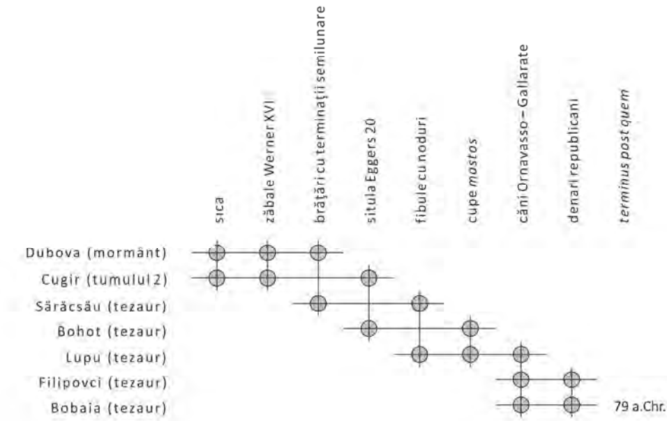
Figura 1. Relații asociative între tipuri reprezentative din câteva inventare diagnostic de epocă târzie La Tène de la Dunărea de Jos și din Transilvania / Correspondence relationships between representative types from Late La Tène diagnostic inventories (graves and hoards) in Transylvania and Lower Danube.
