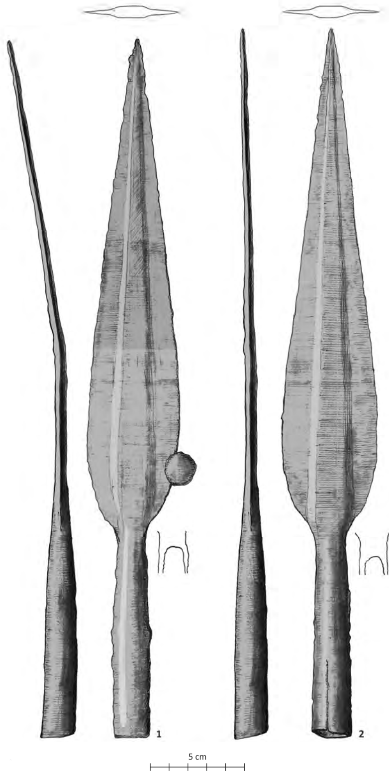
Figura 10. Vârfurile de lance din complexul 4/2019 (desene D. Spânu) / The spearheads from feature 4/2019 (drawings D. Spânu).
