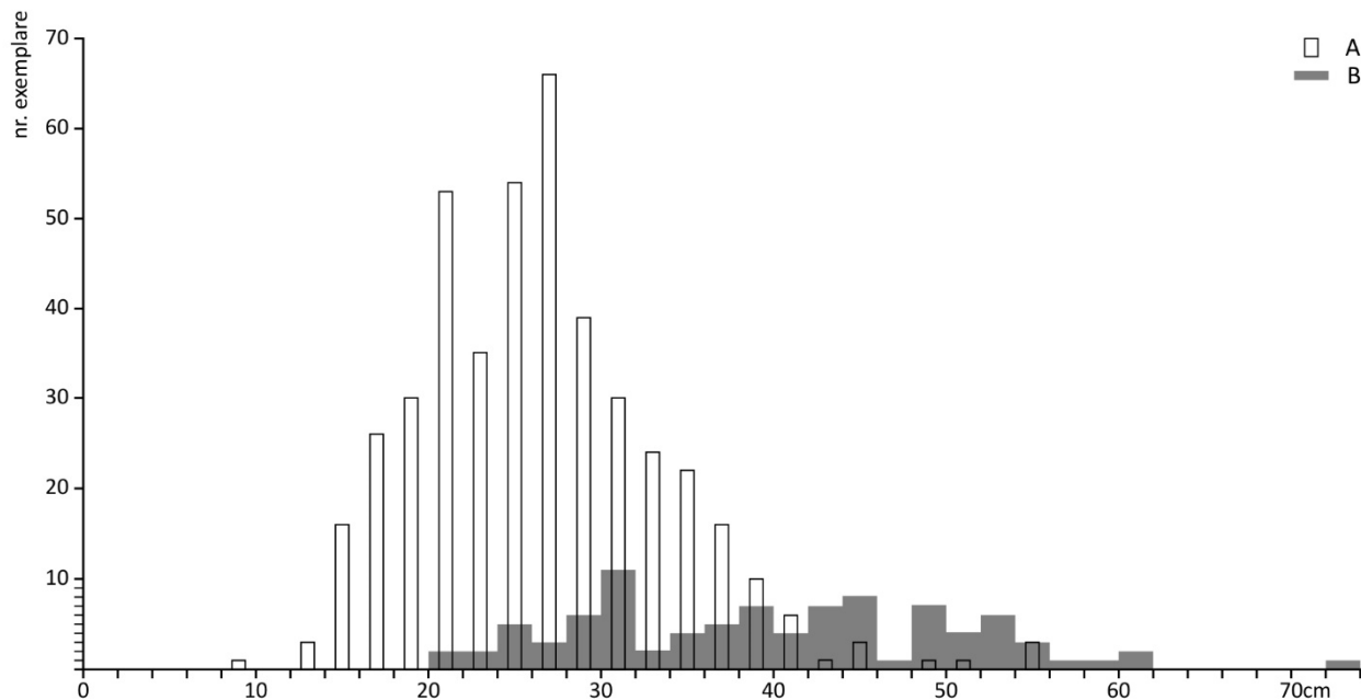
Figura 14. Diagrama lungimilor vârfulor de lance: A. Vârfulor de lance de la Illerup, Nydam și Vimose (după Klimscha et alii 2012, p. 351–353, fig. 1); B. Vârfulor de lance din aria Padea – Panagjurski Kolonii (v. Anexa 2) / Spearhead length diagram: A. spearheads from Illerup, Nydam and Vimose (after Klimscha et alii 2012, p. 351–353, fig. 1); B. Spearheads from Padea – Panagjurski Kolonii contexts (see Appendix 2).
