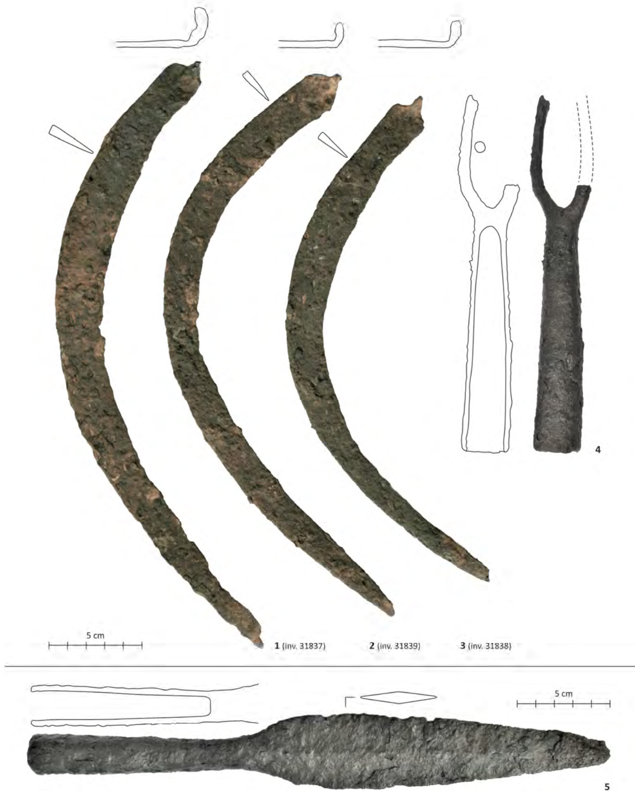
Figura 4. 1–3. Secerile (fotografii și secțiuni D. Spânu); 4. Furca de măcelărie cu tub de înmănușare (fotografie G. Mureșan, desen D. Spânu); 5. Vârful de lance găsit la 400 m de locul de descoperire a depozitului de unelte (fotografie G. Mureșan, secțiuni D. Spânu). 1–5. Fier / 1–3. Iron sickles (photo and cross-sections D. Spânu); 4. Iron socketed flesh fork (photo G. Mureșan, drawing D. Spânu); 5. Iron spearhead discovered at 400 m distance from the tools-deposit (photo G. Mureșan, cross-sections D. Spânu).
