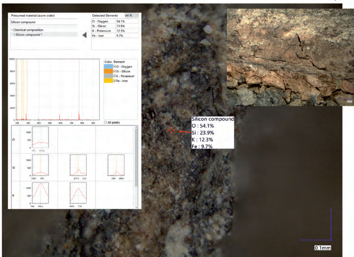
Planşa II. Vasul 1: Reconstruire grafică; Analize microscopice.
